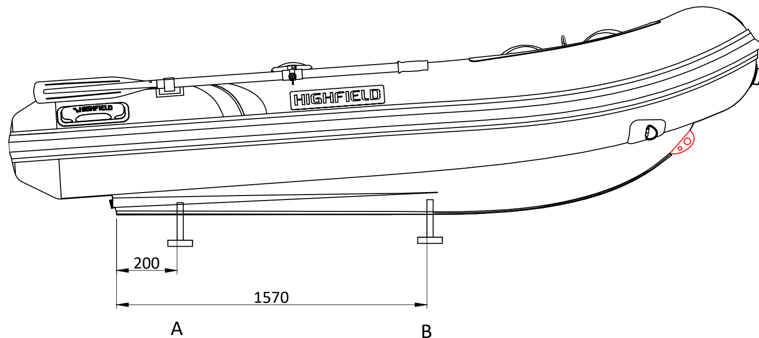
LONGITUDINAL PROFILE
