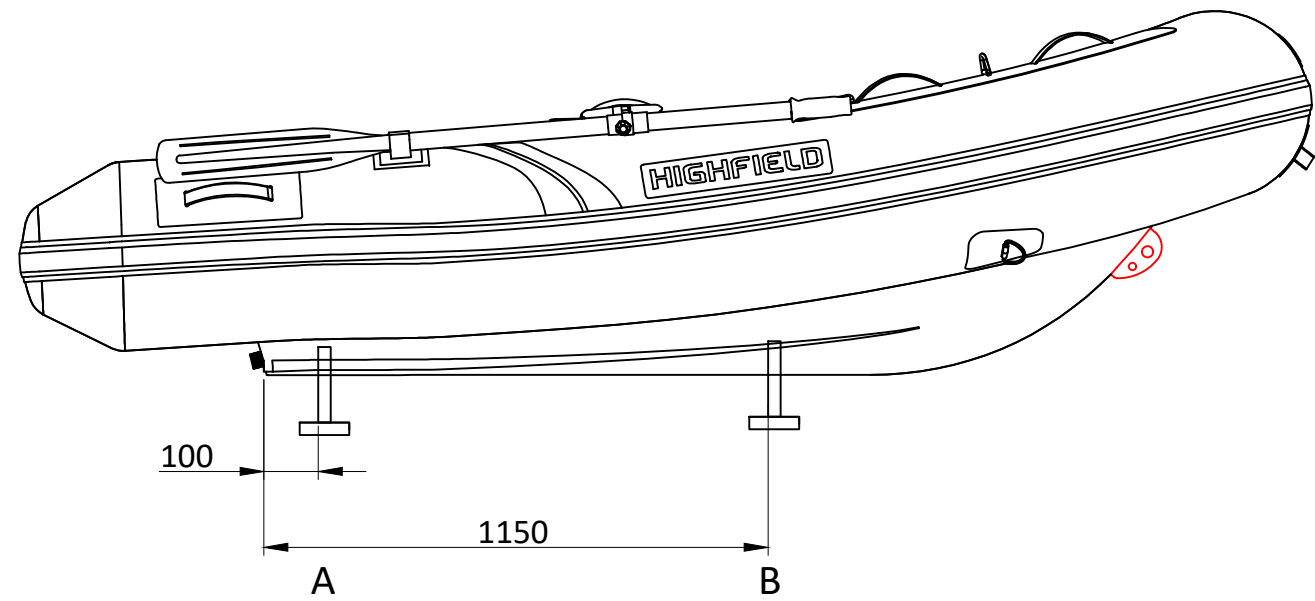
LONGITUDINAL PROFILE
