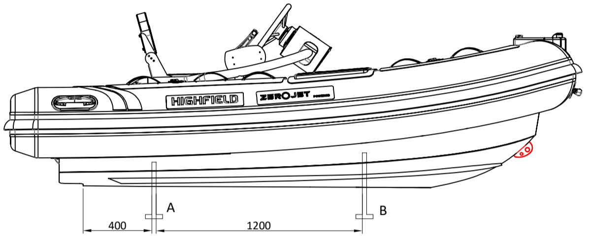
LONGITUDINAL PROFILE
