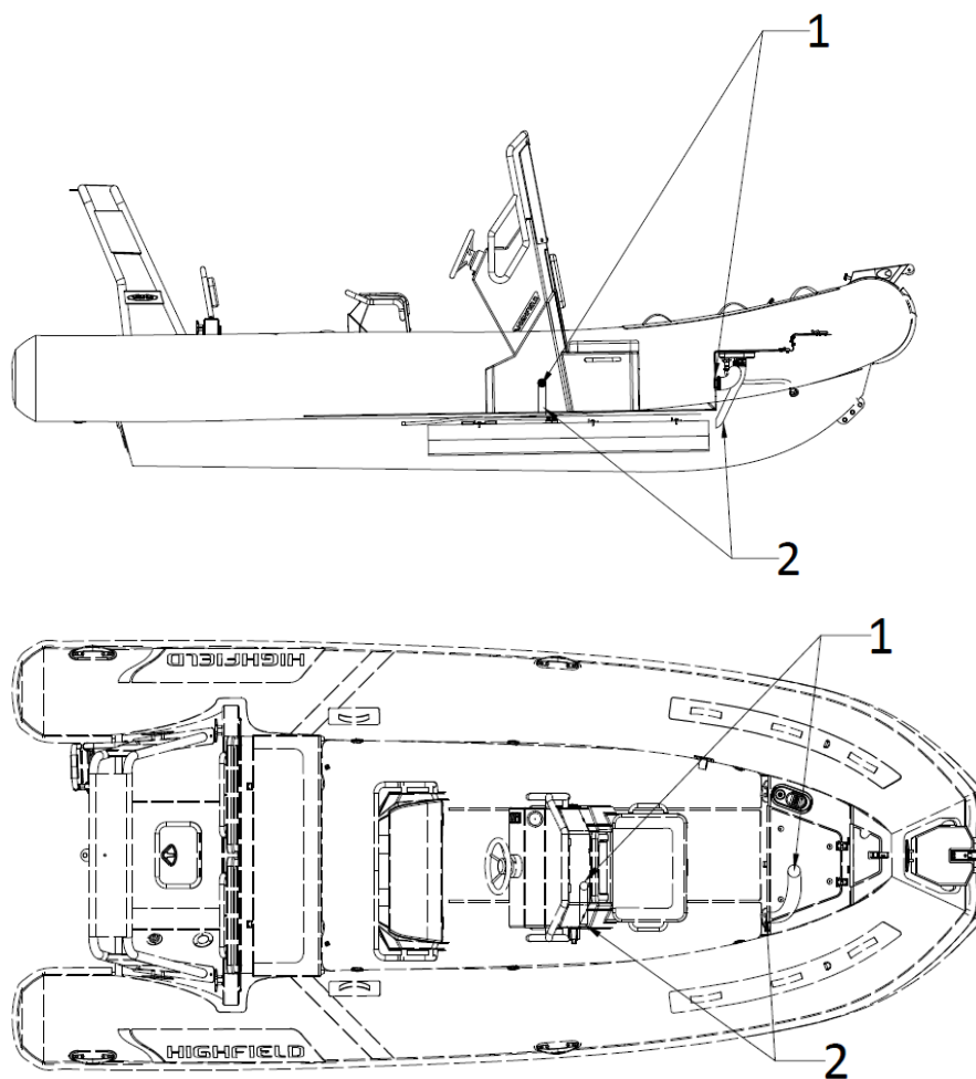
Diagrama del diseño de ventilación del compartimento del depósito de combustible
