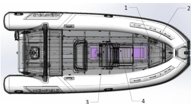
Darstellung Kraftstoffsystem
