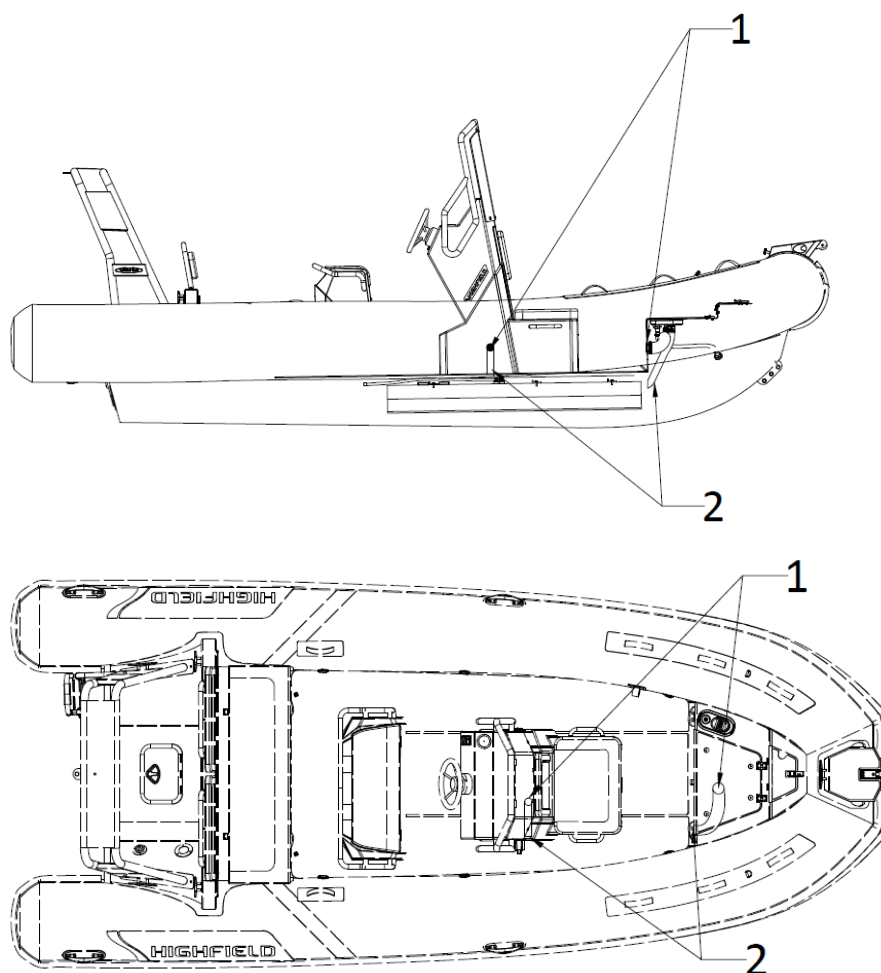
Schéma d'implantation de la ventilation du compartiment du réservoir d'essence.
