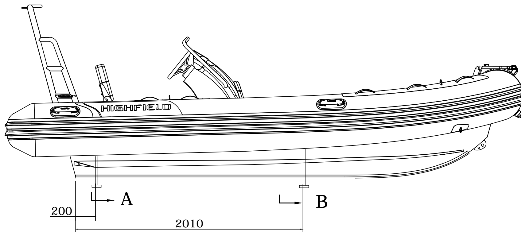
LONGITUDINAL PROFILE
