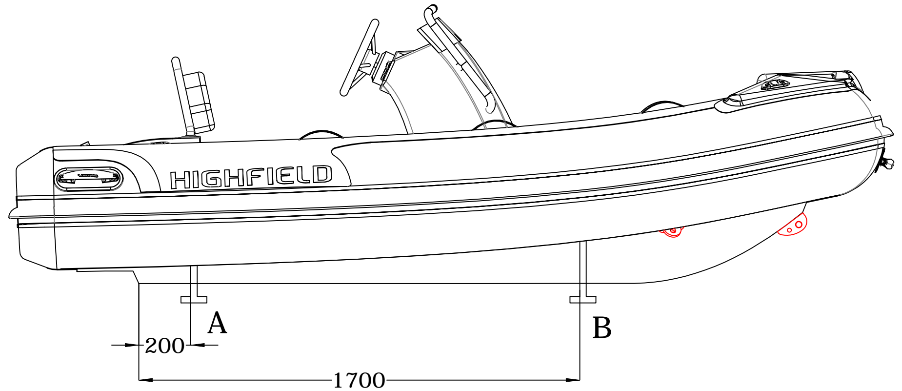
LONGITUDINAL PROFILE
