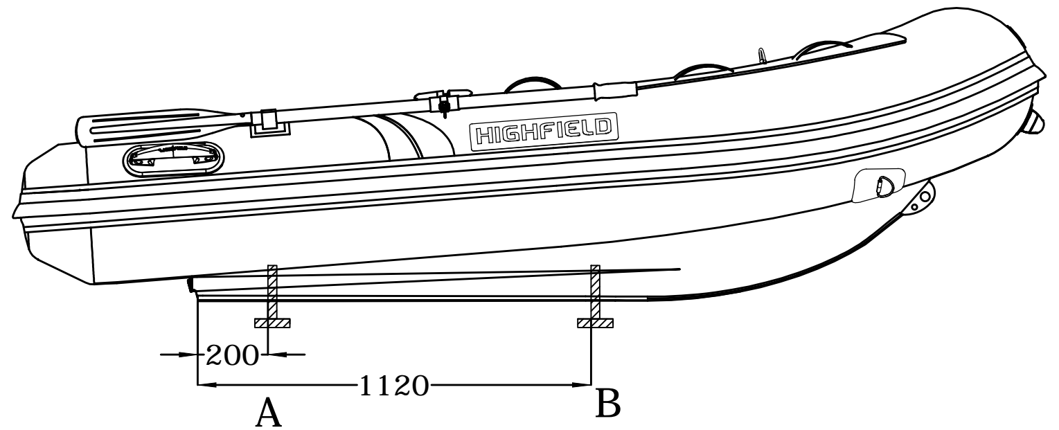
LONGITUDINAL PROFILE
