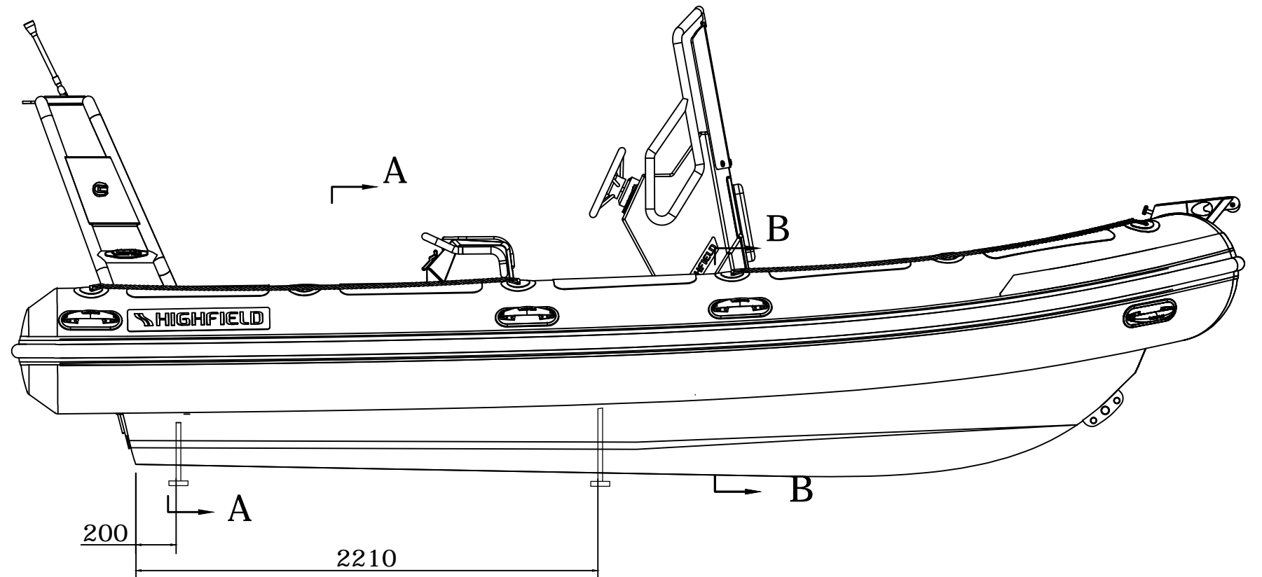
LONGITUDINAL PROFILE
