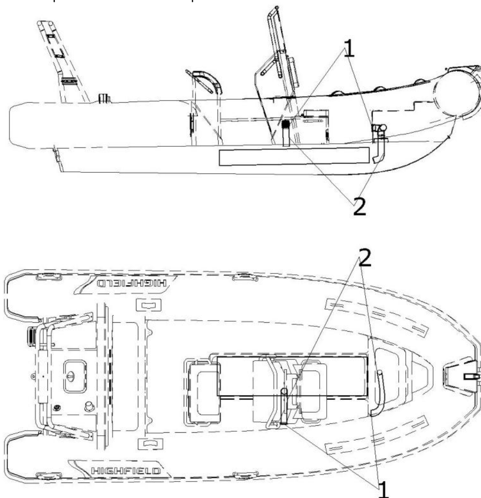
Schéma d'implantation de la ventilation du compartiment du réservoir d'essence.
