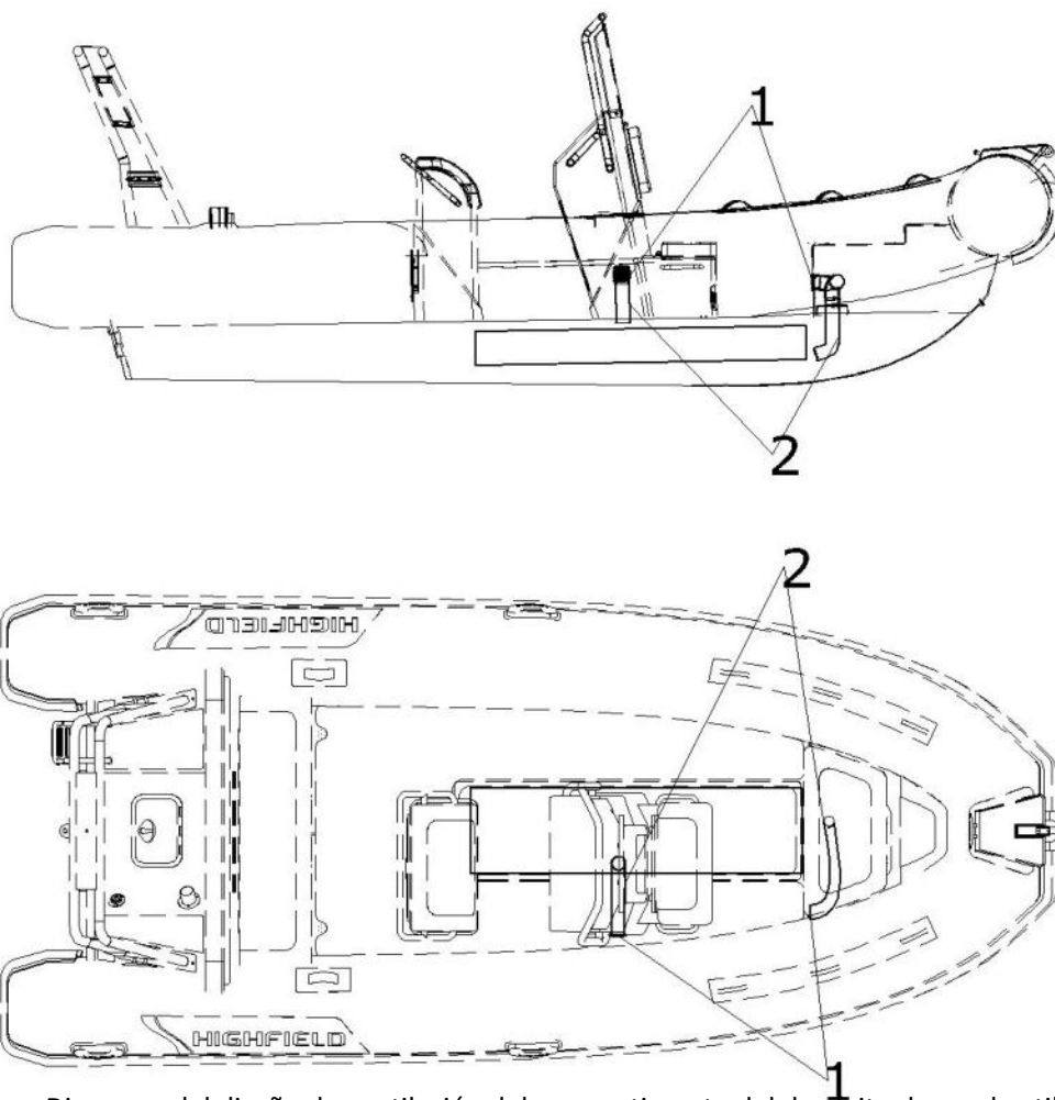
Diagrama del diseño de ventilación del compartimento del depósito de combustible
