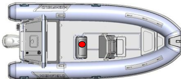
Position de l'extincteur portatif
