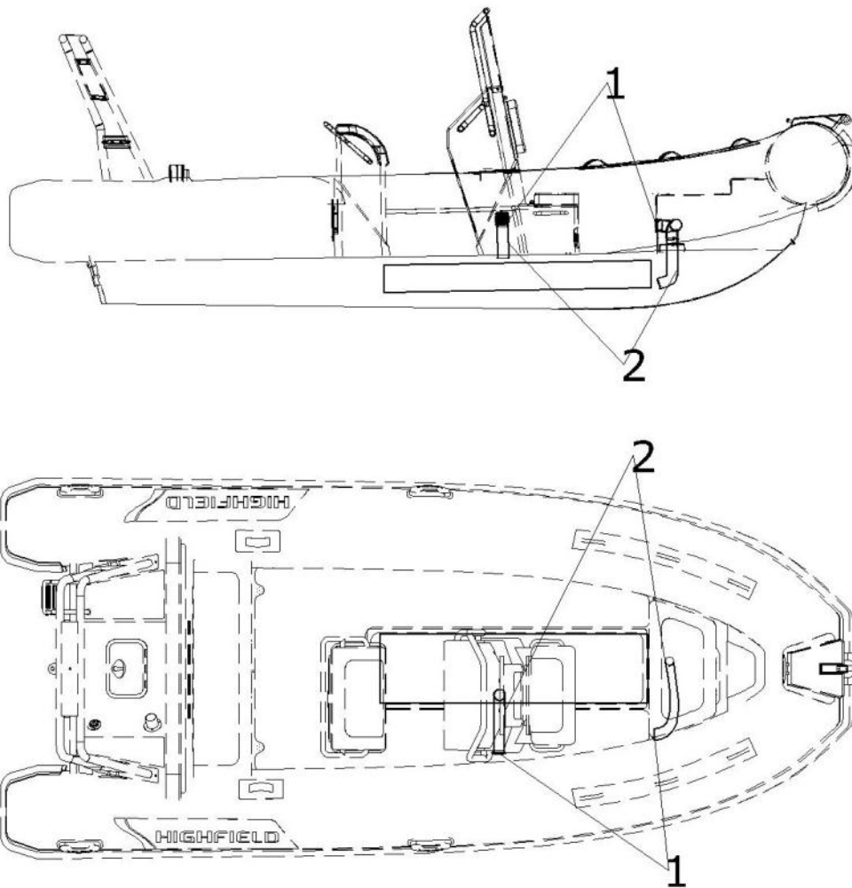
Darstellung der Tankraumbelüftung
