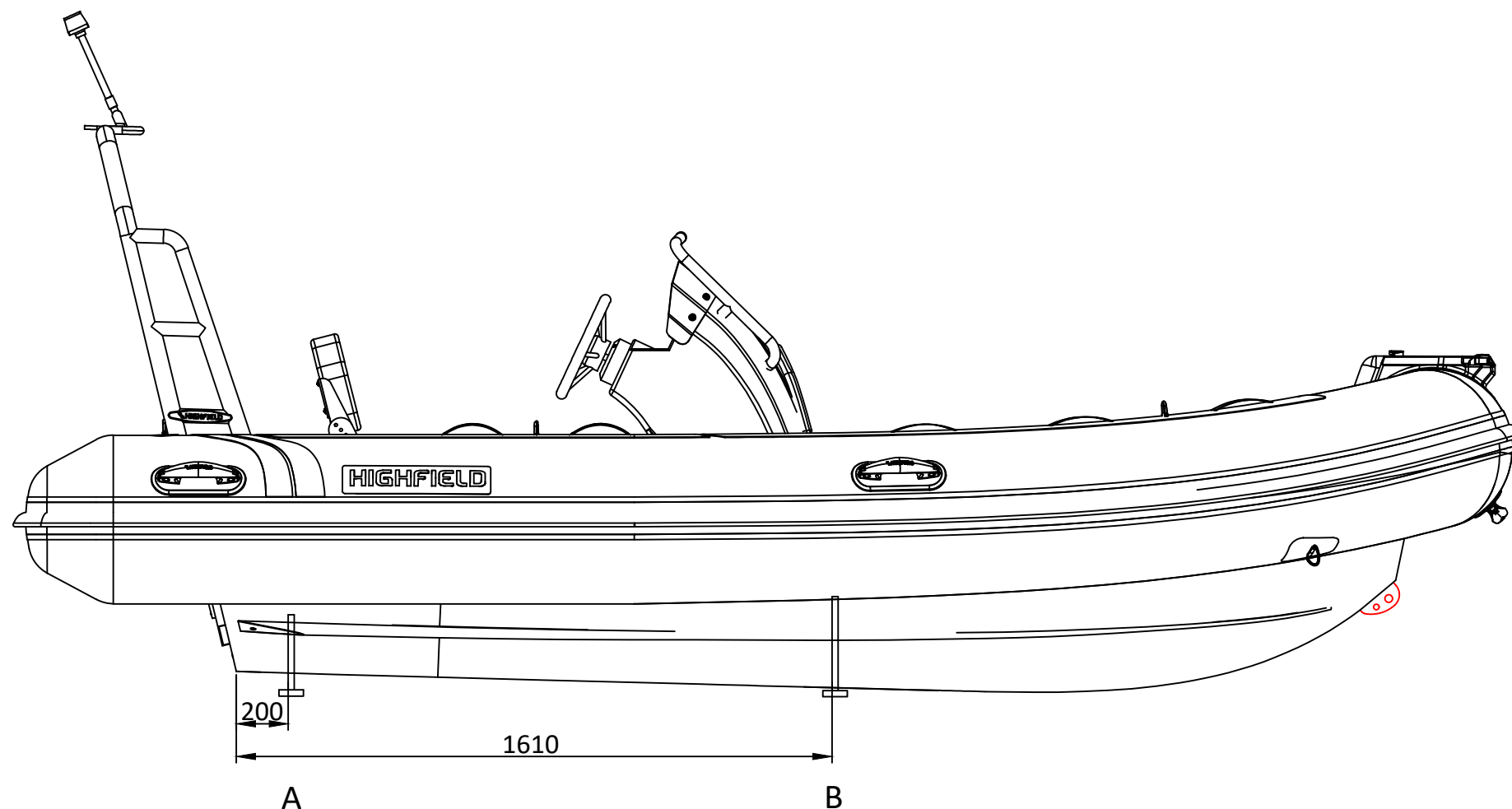
LONGITUDINAL PROFILE
