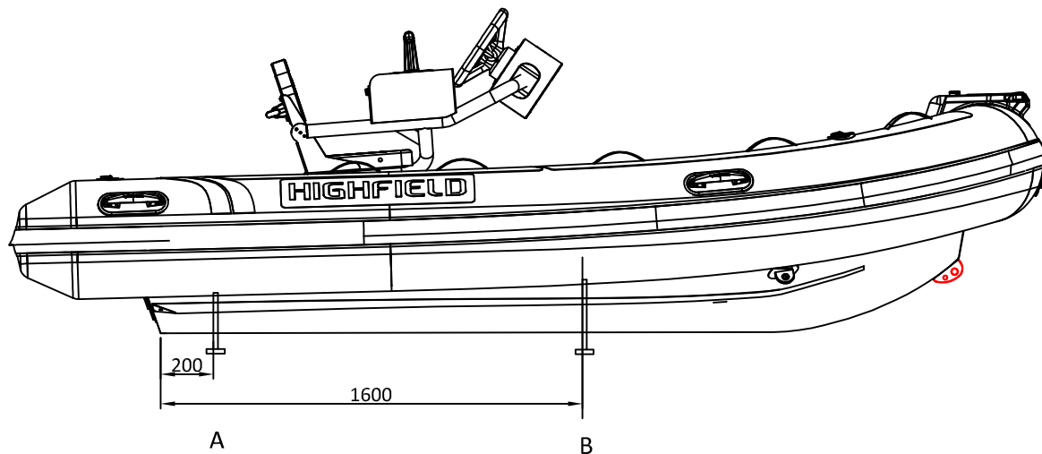
LONGITUDINAL PROFILE
