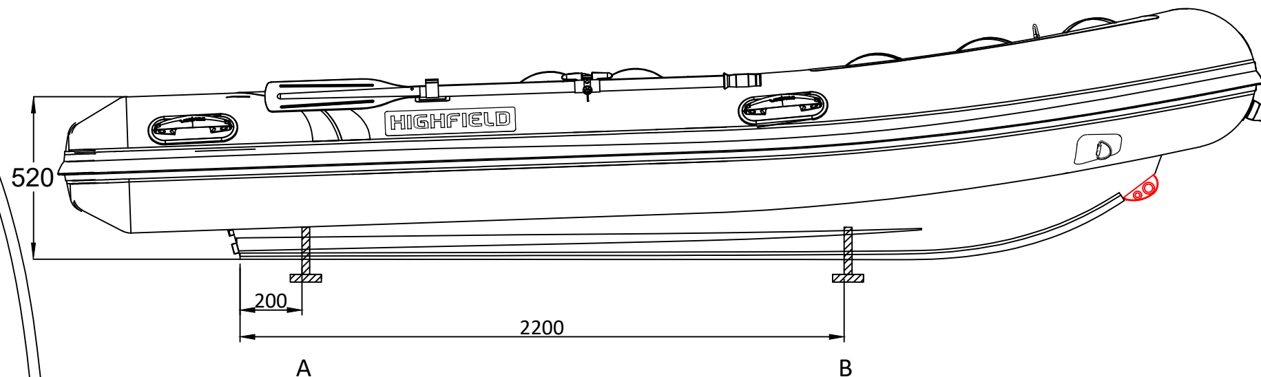
LONGITUDINAL PROFILE
