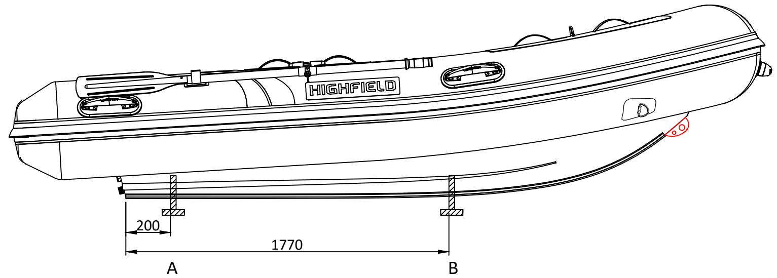
LONGITUDINAL PROFILE
