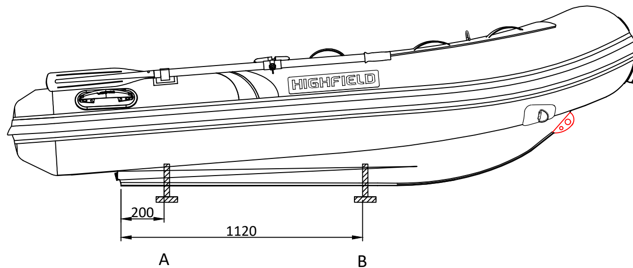
LONGITUDINAL PROFILE
