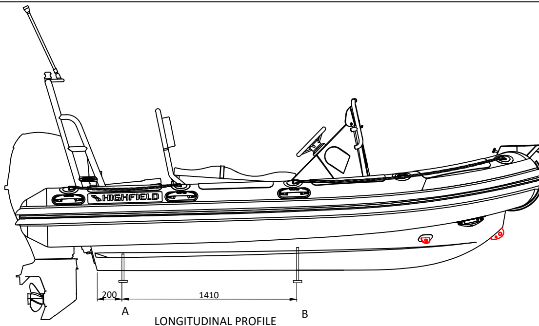
LONGITUDINAL PROFILE
