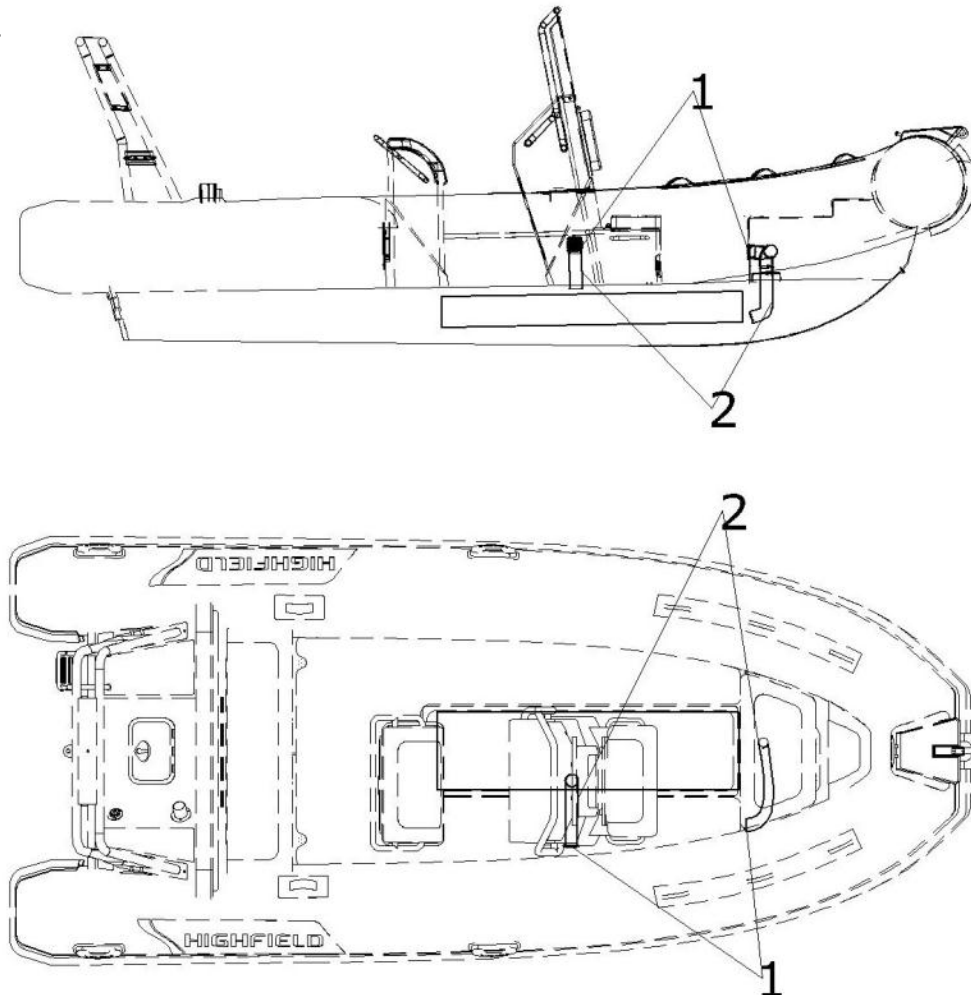
Schéma d'implantation de la ventilation du compartiment du réservoir d'essence.
