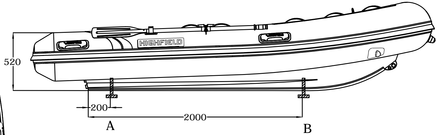
LONGITUDINAL PROFILE
