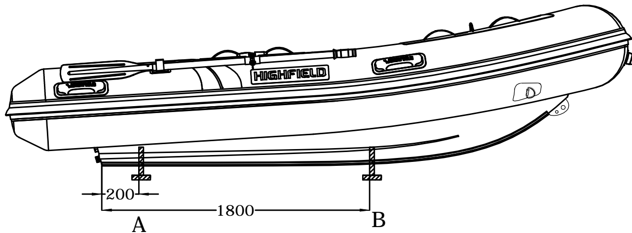
LONGITUDINAL PROFILE
