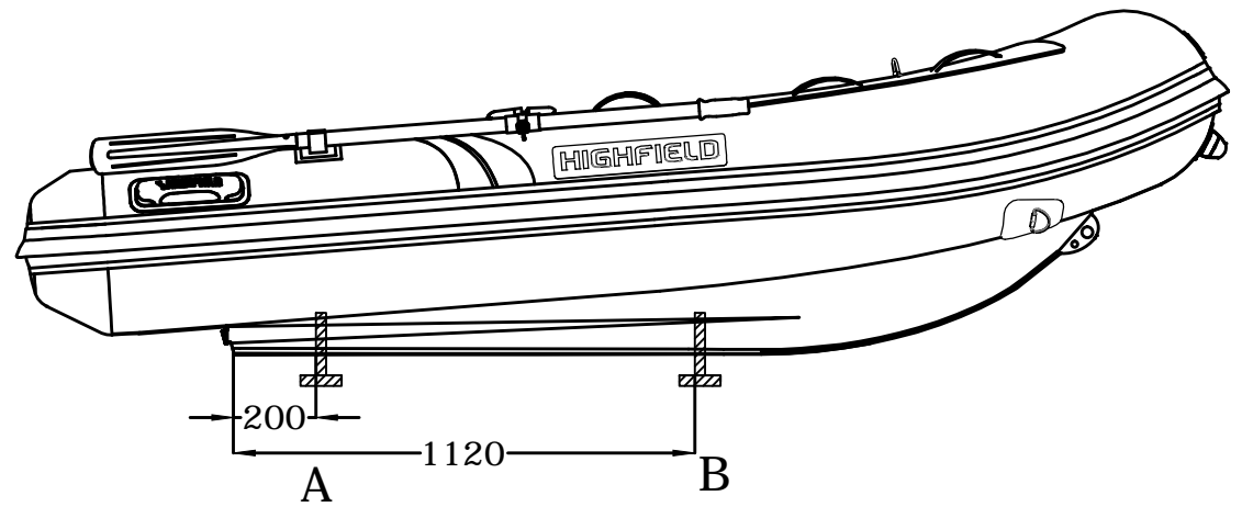
LONGITUDINAL PROFILE
