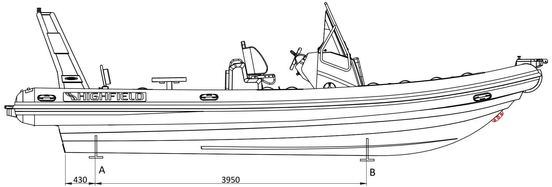
LONGITUDINAL PROFILE
