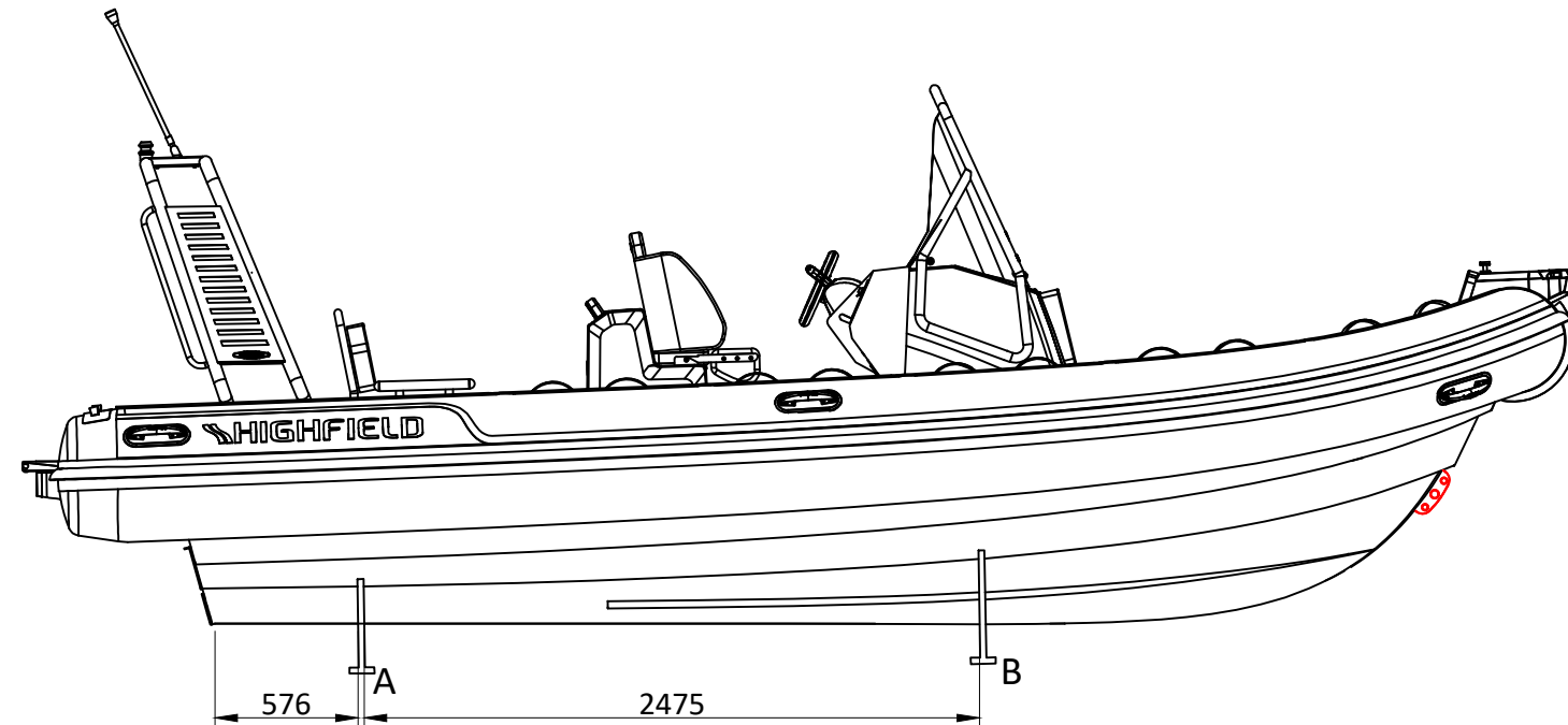
LONGITUDINAL PROFILE
