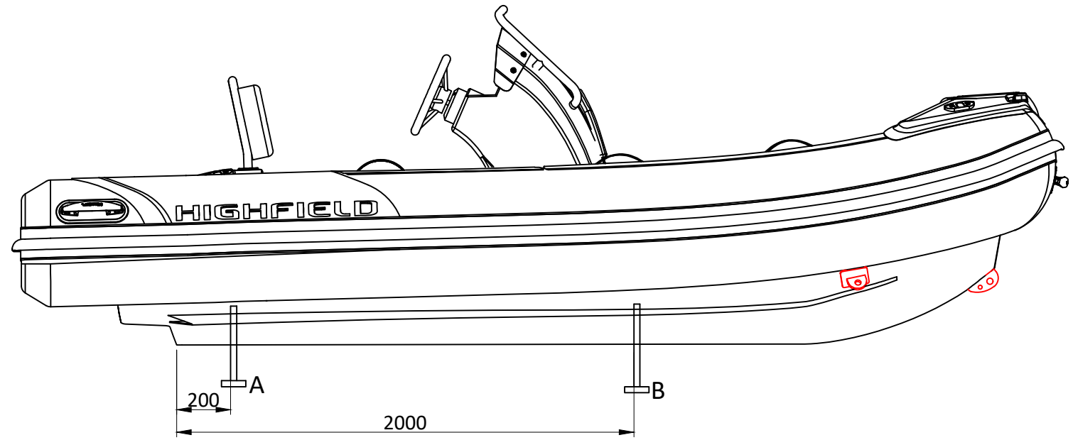
LONGITUDINAL PROFILE
