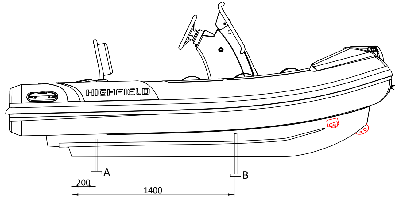
LONGITUDINAL PROFILE
