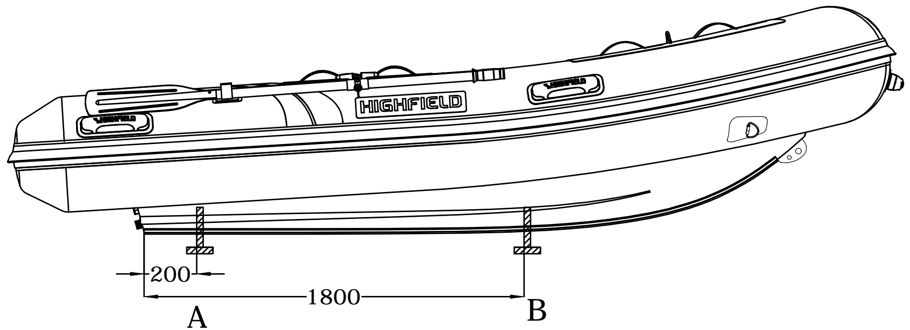
LONGITUDINAL PROFILE
