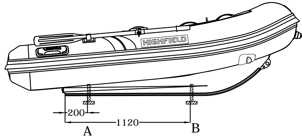
LONGITUDINAL PROFILE
