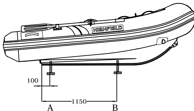
LONGITUDINAL PROFILE
