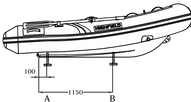
LONGITUDINAL PROFILE
