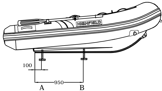
LONGITUDINAL PROFILE
