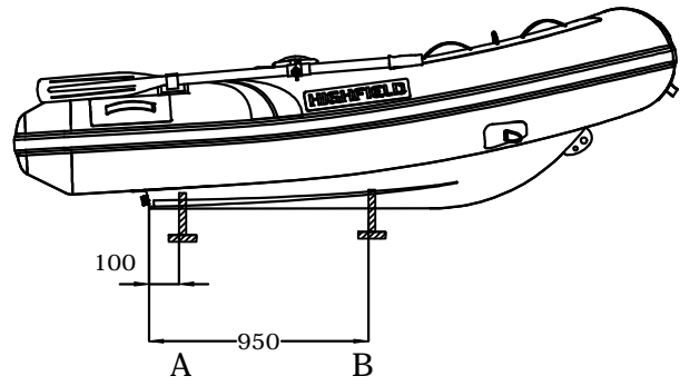
LONGITUDINAL PROFILE
