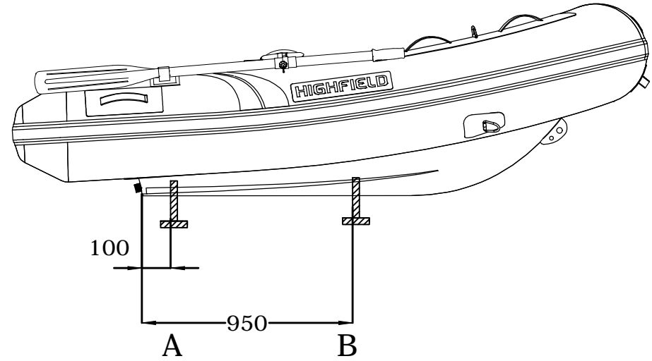
LONGITUDINAL PROFILE
